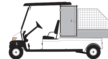
A1H2+ TWIN + RIDELLES GRILLAGÉES
